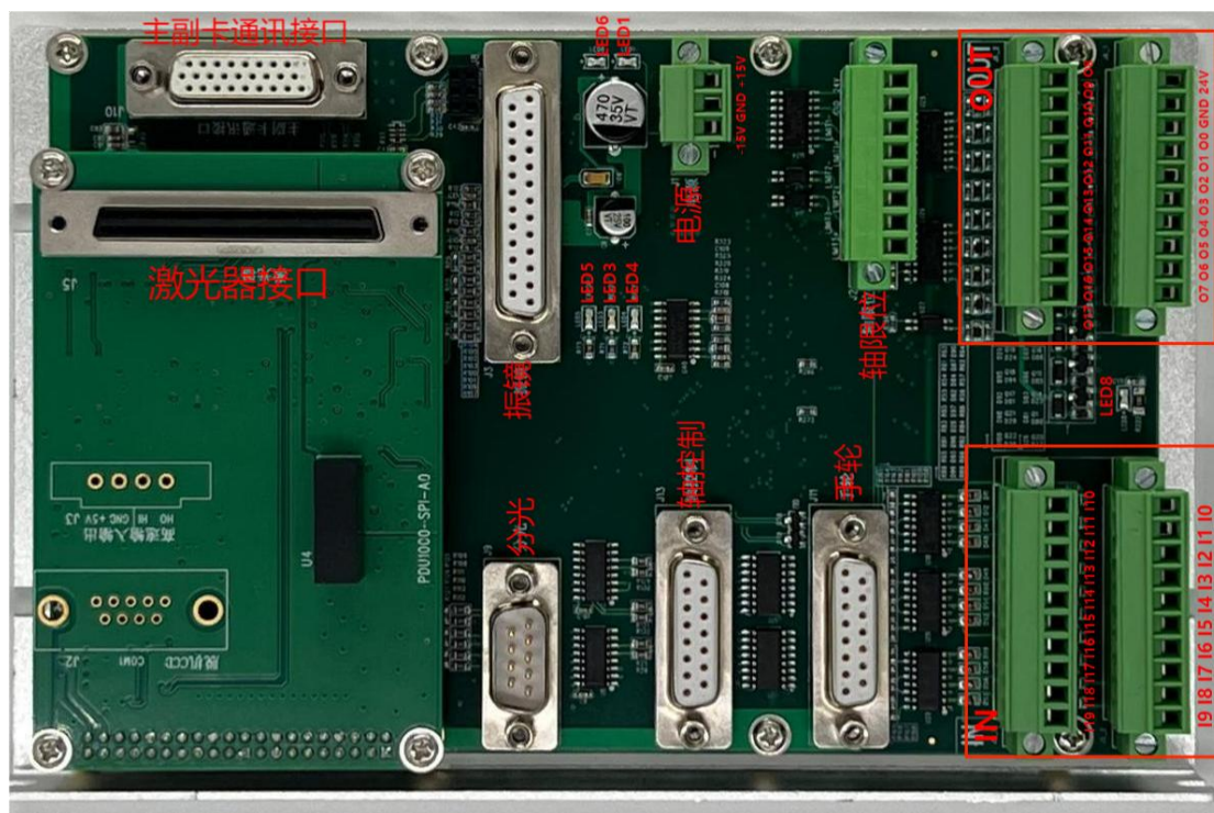
PCIE 端子板
